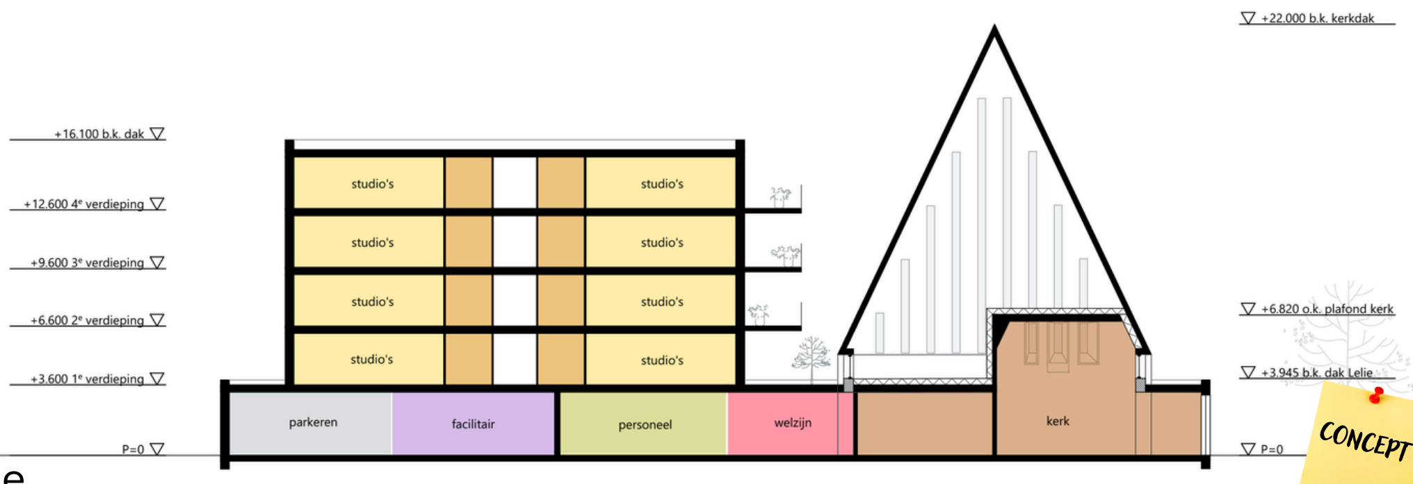
Begane grond
